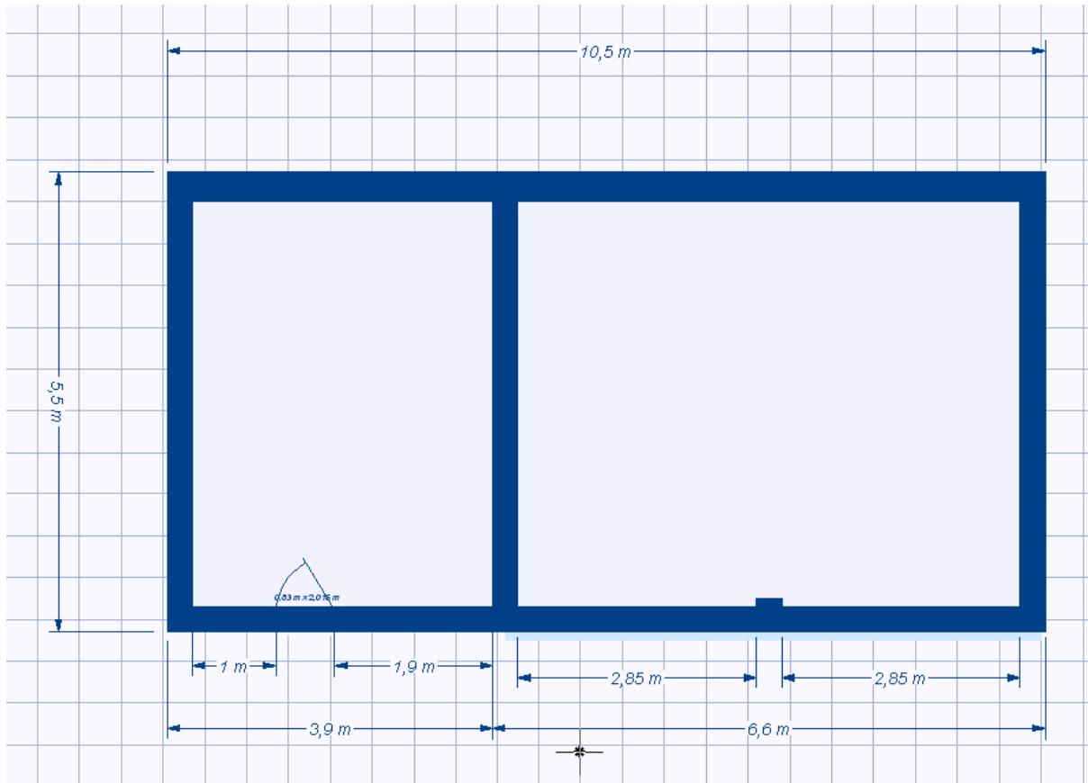
Figure 6 : Vue en coupe de dessus
